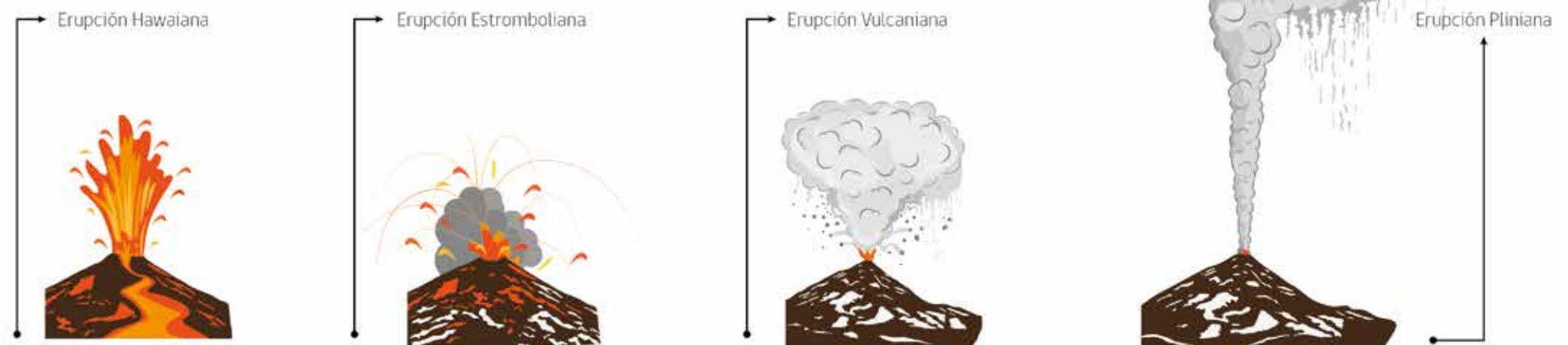
Figura 6. Tipos de erupciones volcánicas.
