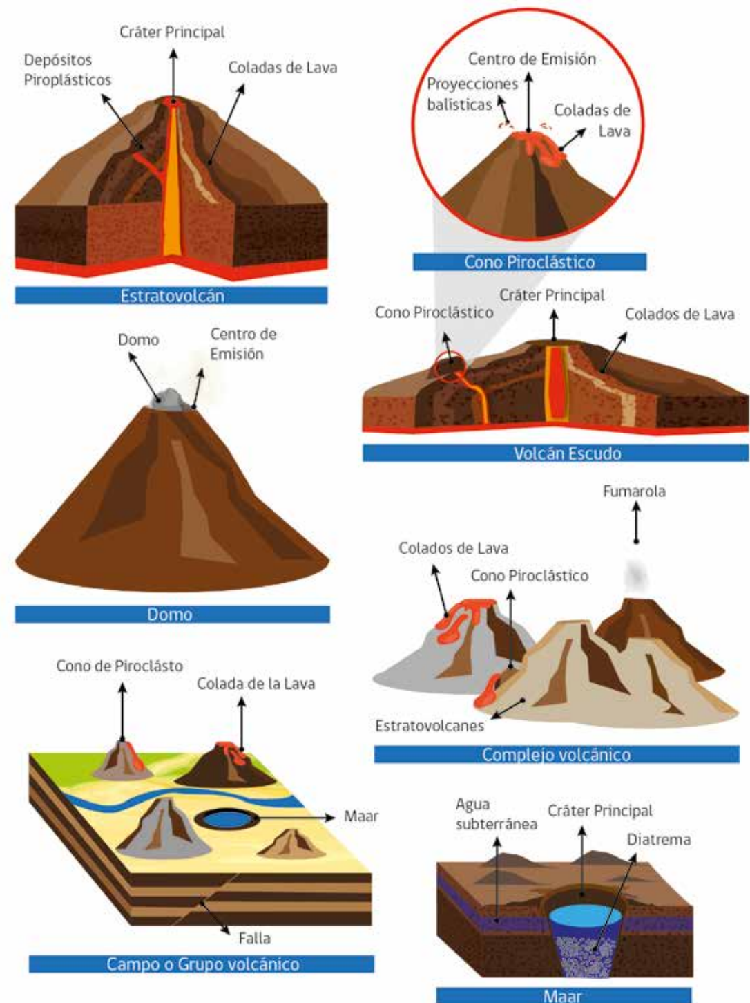
Figura 3. Esquema tipos de volcanes
