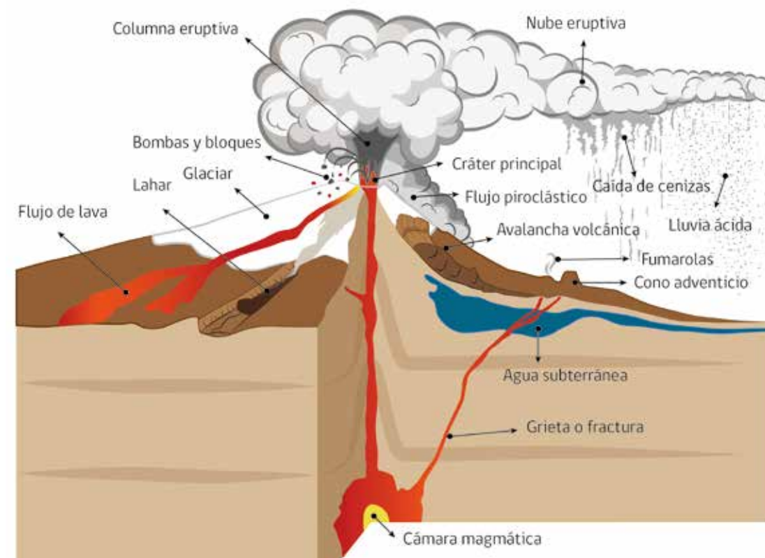
Figura 4. Esquema sobre procesos volcánicos.
