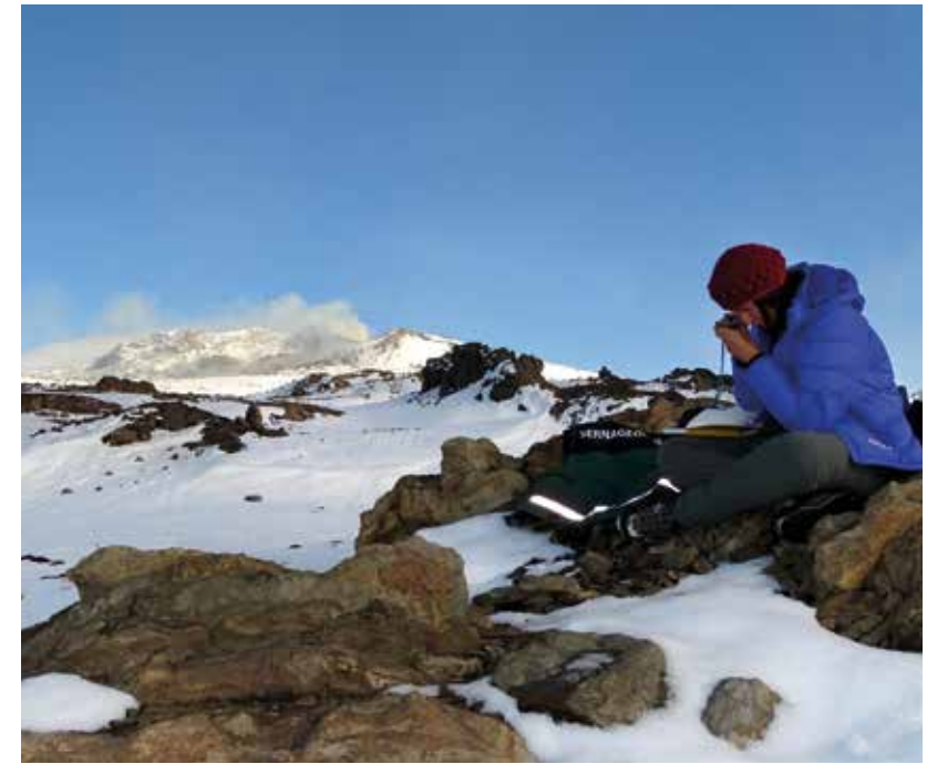
Foto 1. Depósito de caída piroclástica 2011, Complejo volcánico Puyehue-Cordón Caulle. Autor: Álvaro Amigo Ramos. | Foto 2. Secuencia de caída piroclástica, Complejo volcánico Nevados de Chillán. Autor: Sernageomin. | Foto 3. Volcán Copahue. Autor: Felipe Flores Lobos.
