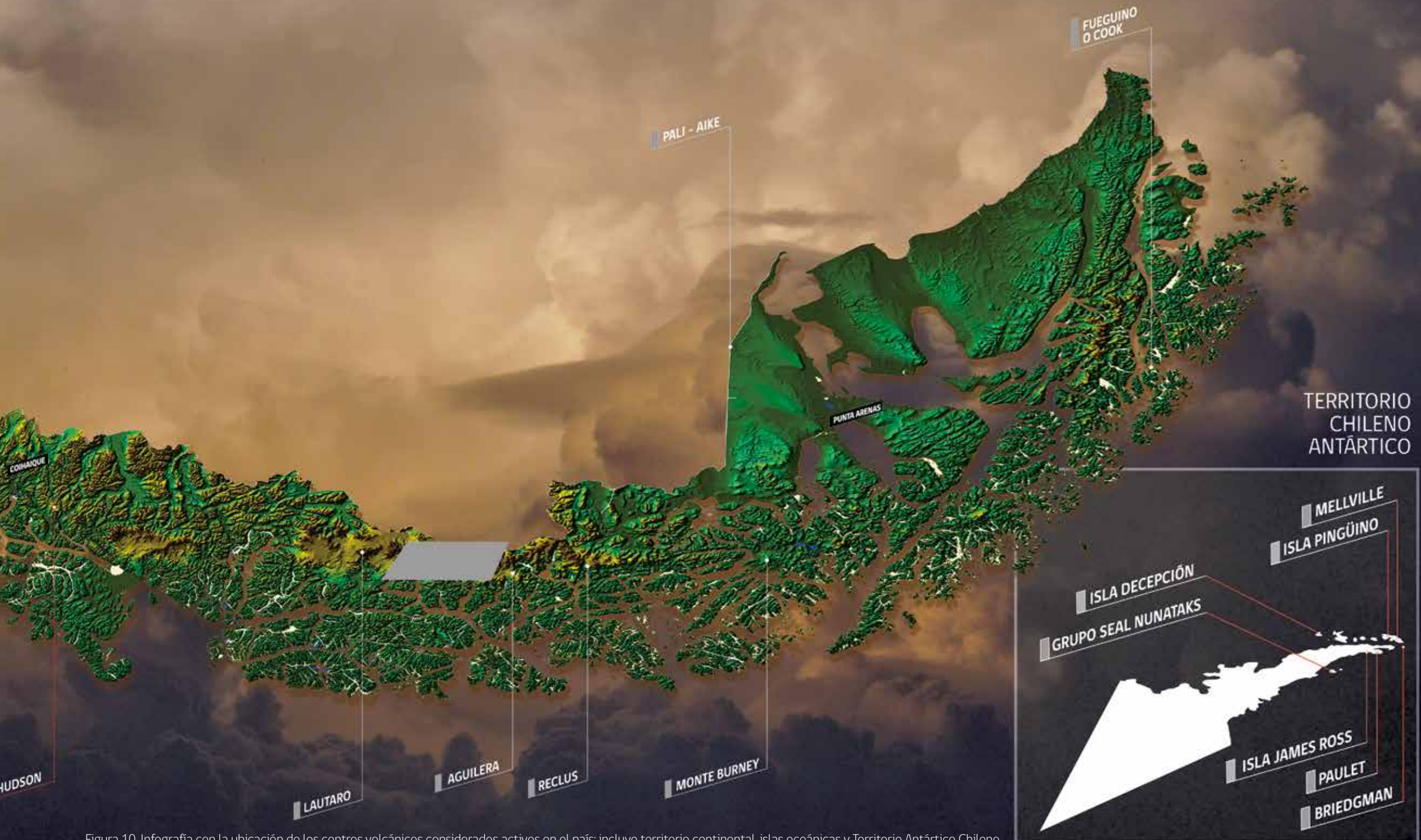
Figura 10. Infografía con la ubicación de los centros volcánicos considerados activos en el país; incluye territorio continental, islas oceánicas y Territorio Antártico Chileno.
