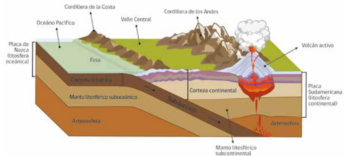
Figura 2. Proceso de subducción de placas tectónicas, lo cual refleja el caso de Chile continental.
