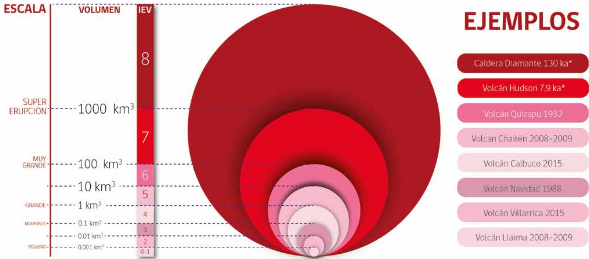
Figura 5. Escala que muestra la clasificación de magnitud eruptiva a través del Índice de Explosividad Volcánica (IEV). En volumen se considera solo material piroclástico emitido; esto excluye volumen eruptivo asociado a lavas.
