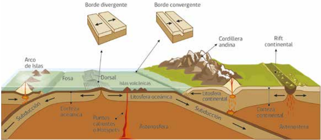
Figura 1. Diferentes ambientes geológicos donde se genera volcanismo.
