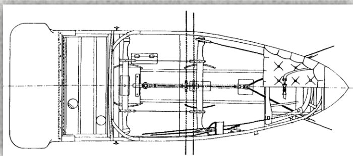
Detalle de la carlinga vista lateral y superior
