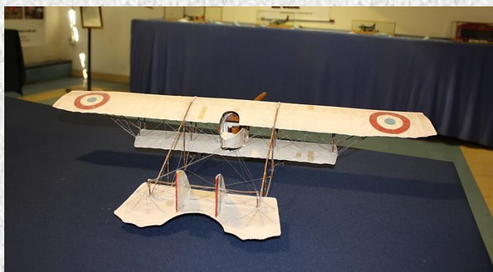
Maqueta preservada por el Museo Nacional de Aeronáutica de la República Argentina 55
