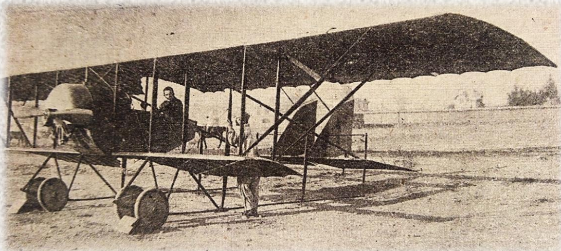
El Caudron G-3 de 80 H.P. ahora de la Sociedad Nacional de Aviación, adquirido por el entusiasta admirador de la aviación, Diógenes Valenzuela Olivos, al representante de Mlle. Bolland, el mecánico Mutt.
